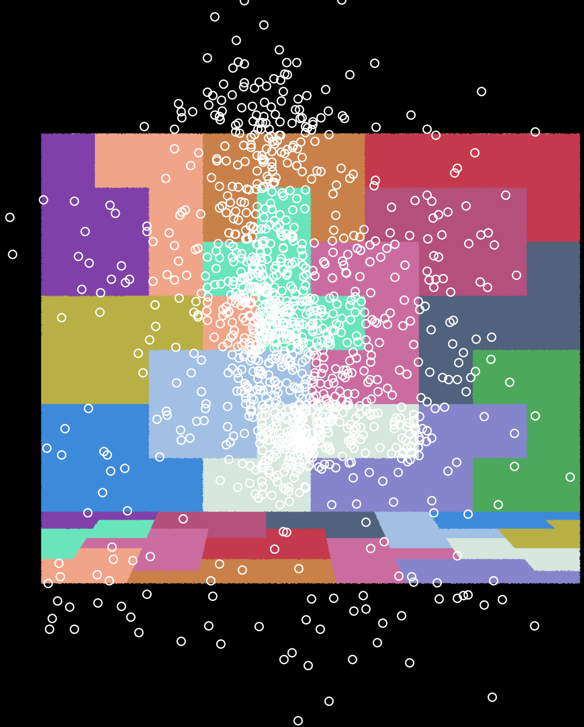
dtmFixedTarget
